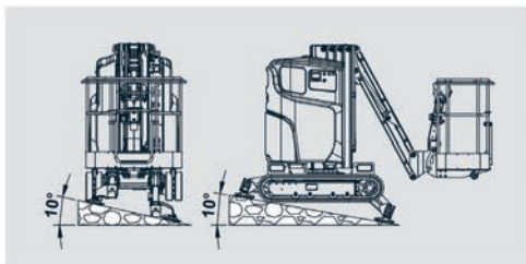
Max. hoek voor zelfstabilisator
