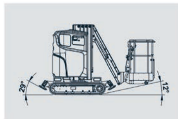
Vrije JIB bij ingeklapte machine
